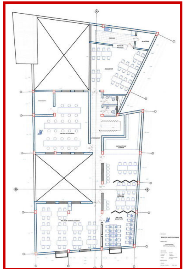
1ª verdieping
